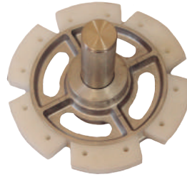
ALUMINIO RUEDA GUIA/TRACCIÓN 300MM PASO 2 RODA GUIA/TRACÇÃO 300MM PASSO 2
