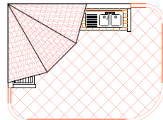
PLANTA CUBIERTA —escala 1:50
