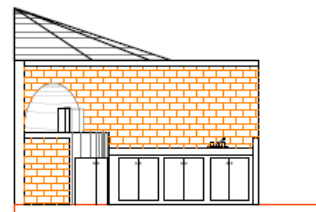
FACHADA FRONTAL —escala 1:50
