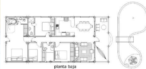
planta baja
