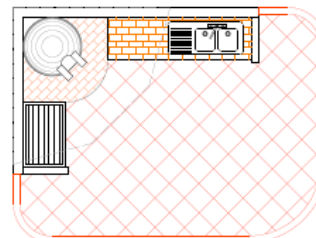
PLANTA N+ 0.15cm —escala 1:50
