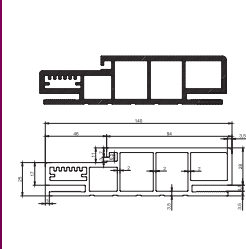
38x75 Pervaz / 38x75 Case
