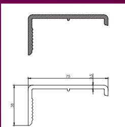
38x75 Pervaz / 38x75 Case
