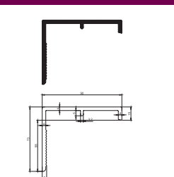
73x90 Pervaz / 73x90 Case
