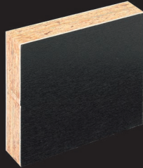
24 mm PVC-OSB-OSB-PVC
